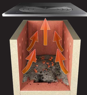
Fase 2: Rilascio del calore dopo la combustione
